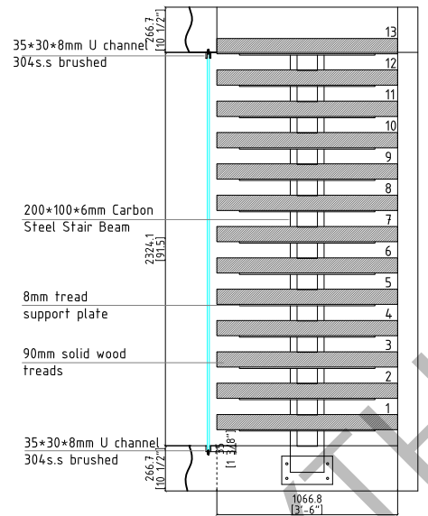
ELEVATION B
